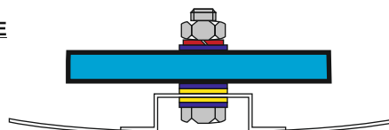
DETAIL SPOJE
